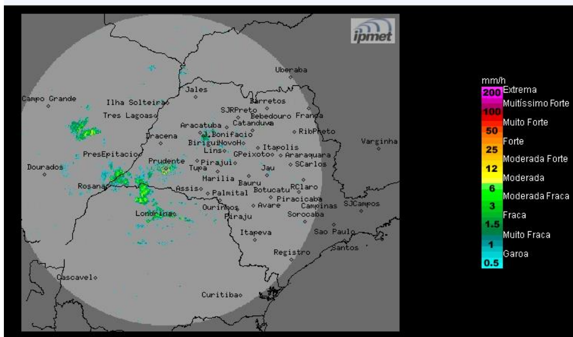
Imagem Composta dos Radares de Bauru e de Presidente Prudente - 24/11/2023 08:30
