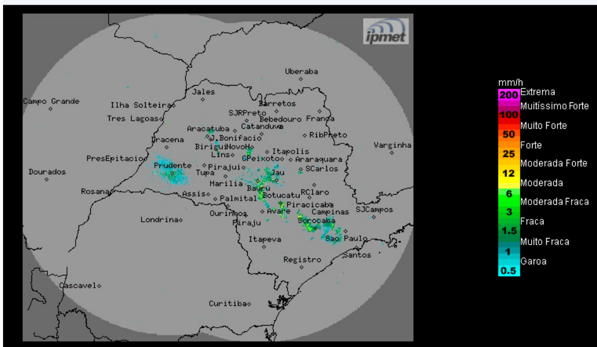
Imagem Composta dos Radares de Bauru e de Presidente Prudente - 27/09/2024 09:30
