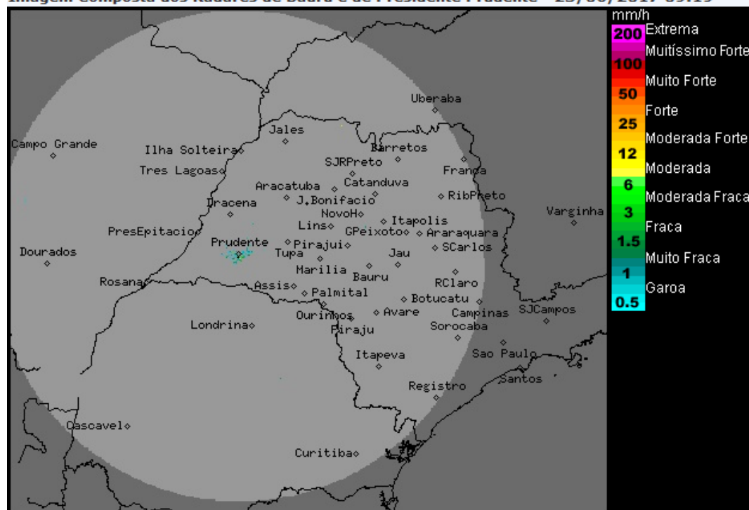
Imagem Composta dos Radares de Bauru e de Presidente Prudente - 23/06/2017 09:19
