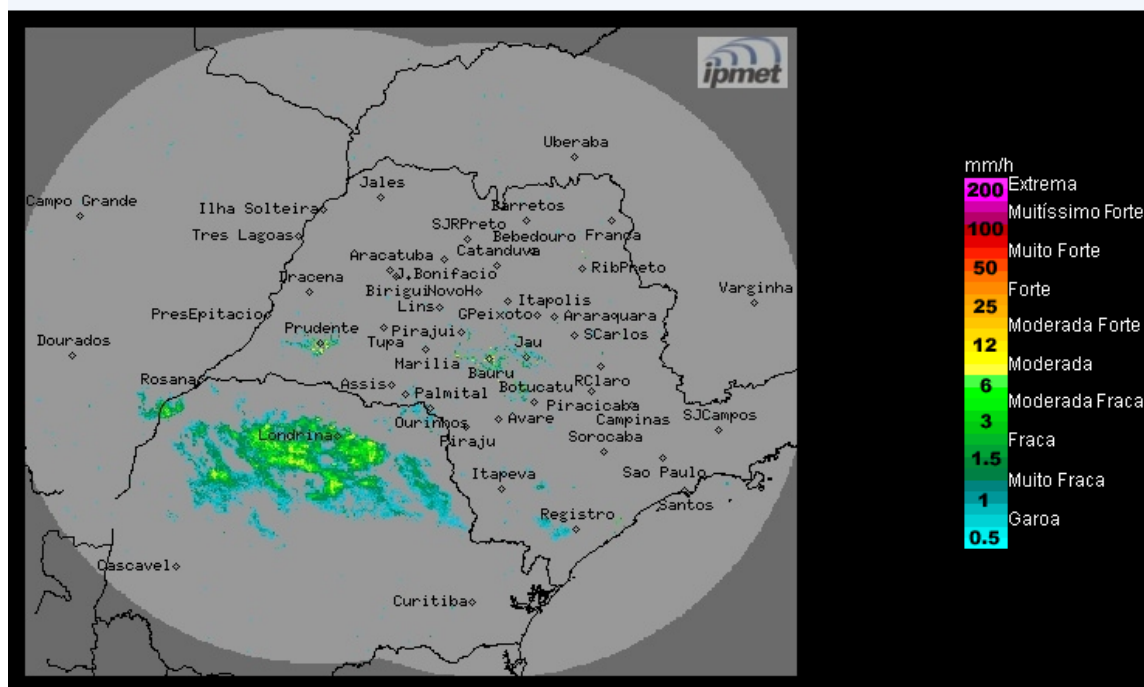
Imagem Composta dos Radares de Bauru e de Presidente Prudente - 16/07/2021 08:30
