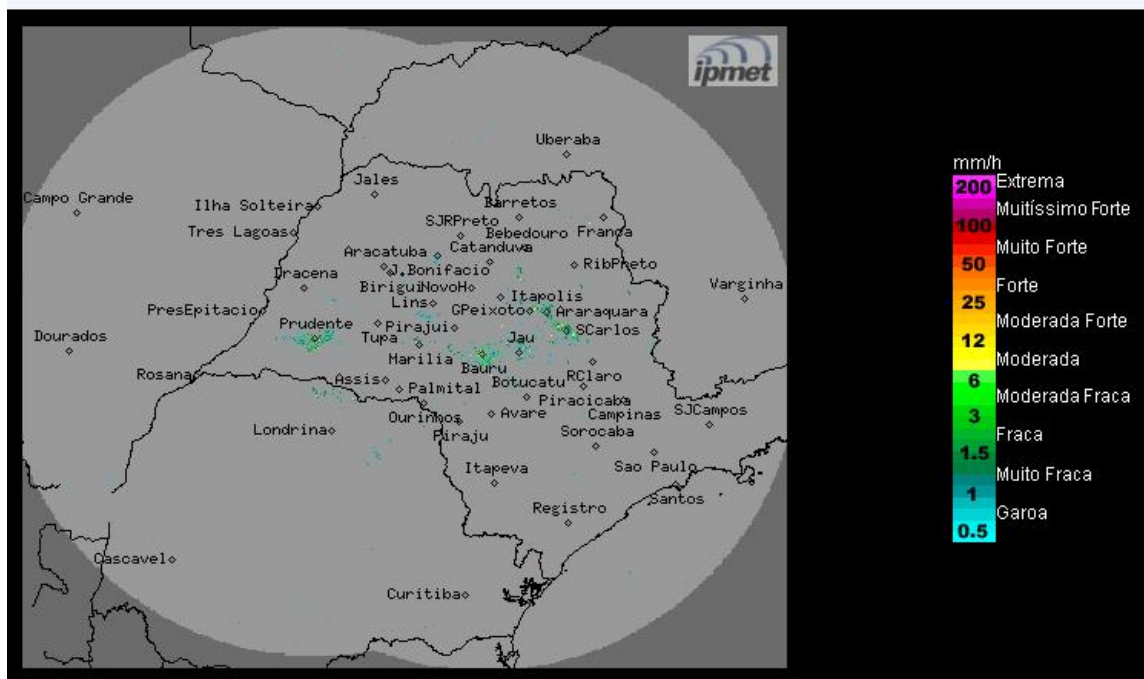
Imagem Composta dos Radares de Bauru e de Presidente Prudente - 22/07/2021 09:00
