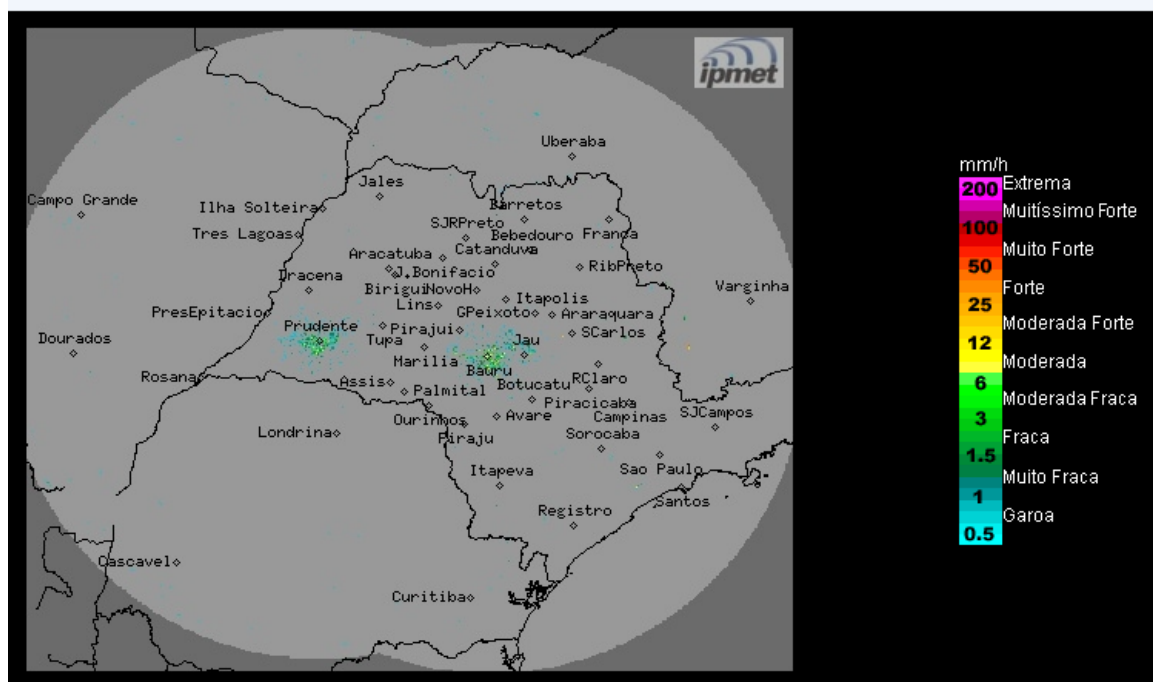
Imagem Composta dos Radares de Bauru e de Presidente Prudente - 04/08/2021 10:00
