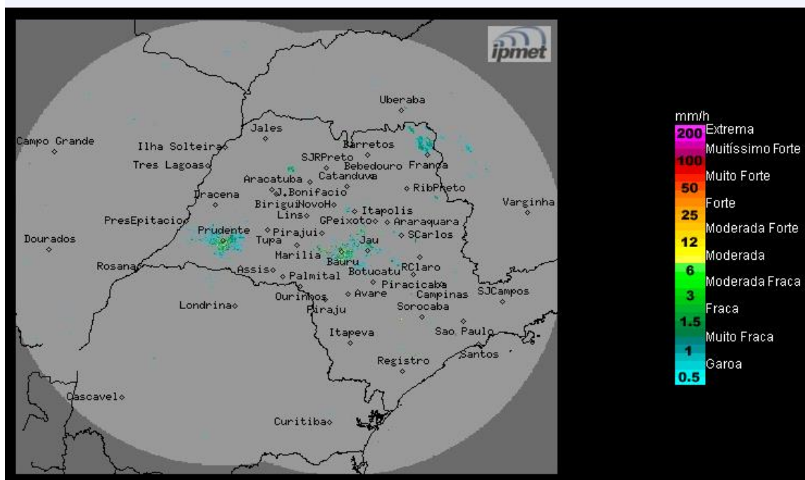
Imagem Composta dos Radares de Bauru e de Presidente Prudente - 26/10/2021 08:15
