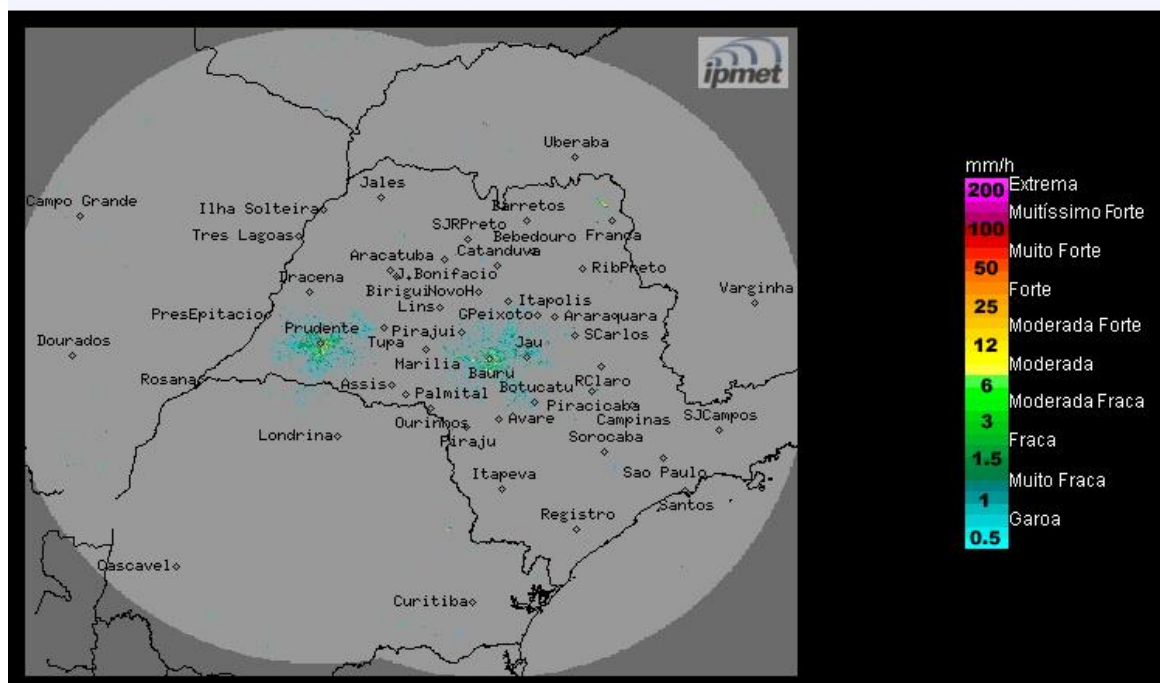
Imagem Composta dos Radares de Bauru e de Presidente Prudente - 22/02/2022 10:00
