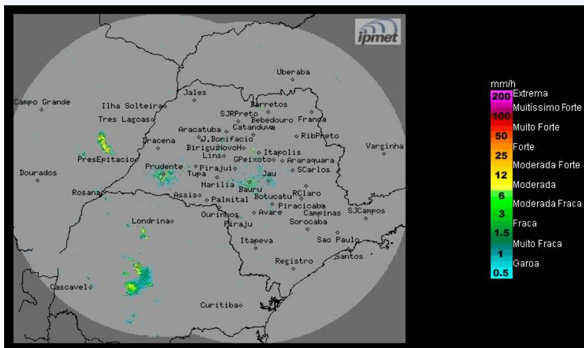
Imagem Composta dos Radares de Bauru e de Presidente Prudente - 30/03/2022 09:37
