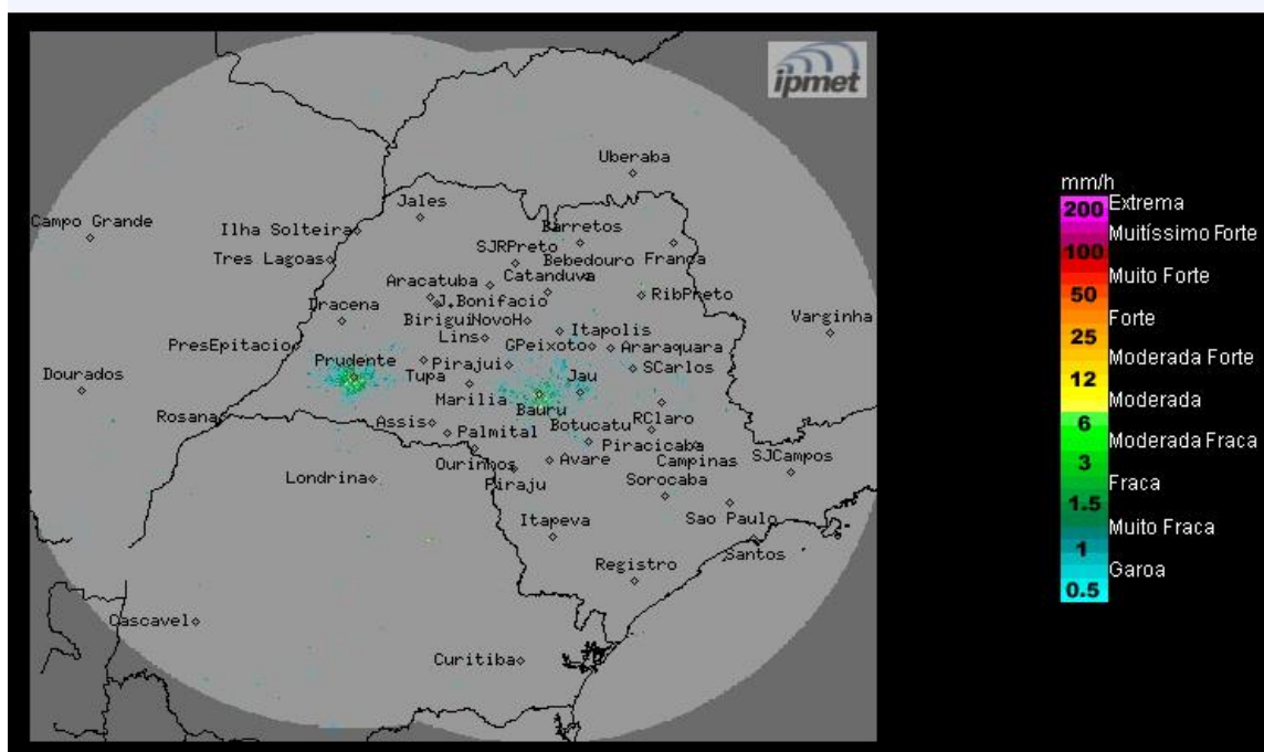
Imagem Composta dos Radares de Bauru e de Presidente Prudente - 05/04/2022 10:00
