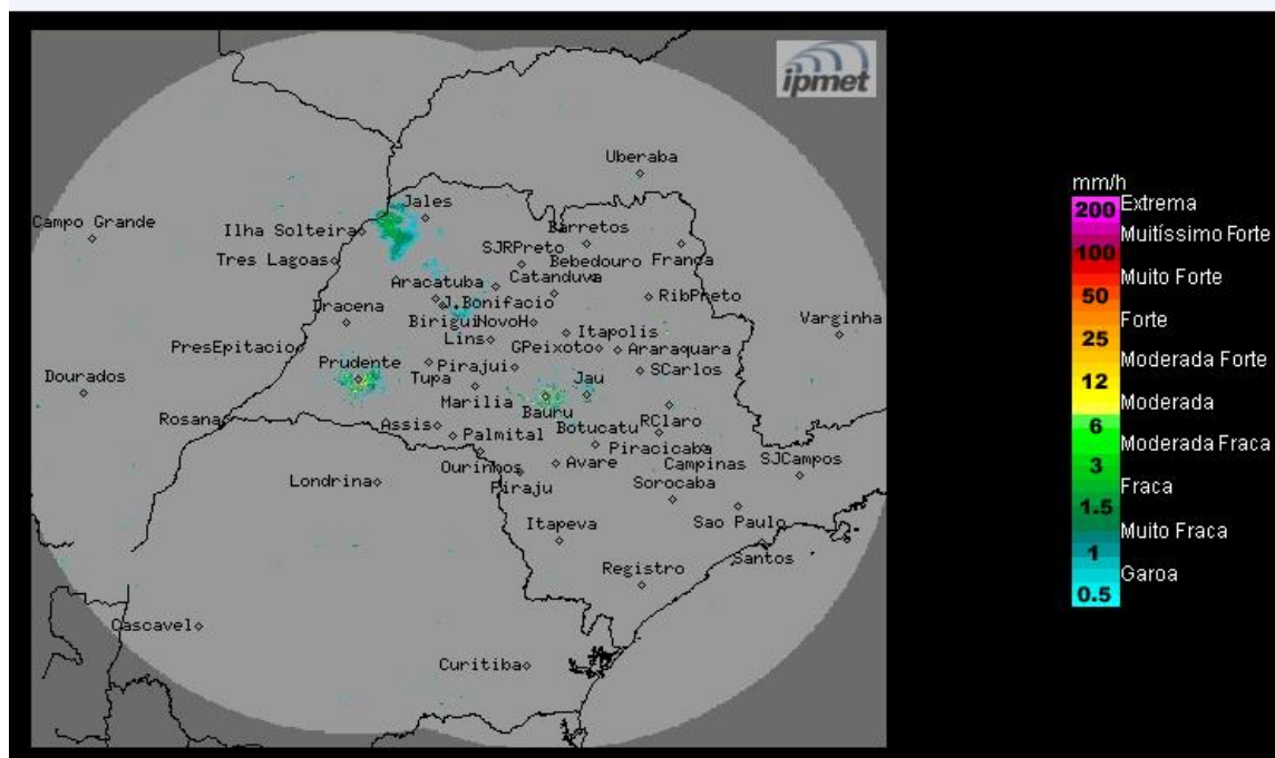
Imagem Composta dos Radares de Bauru e de Presidente Prudente - 08/04/2022 09:15
