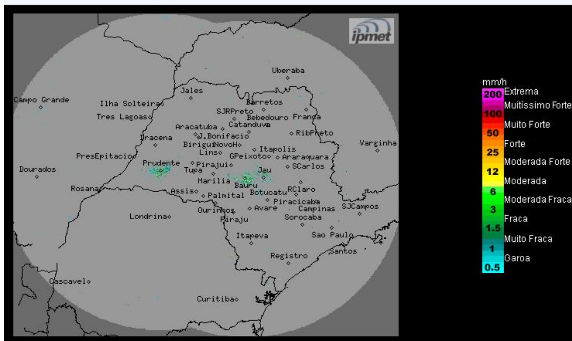
Imagem Composta dos Radares de Bauru e de Presidente Prudente - 27/06/2022 09:00
