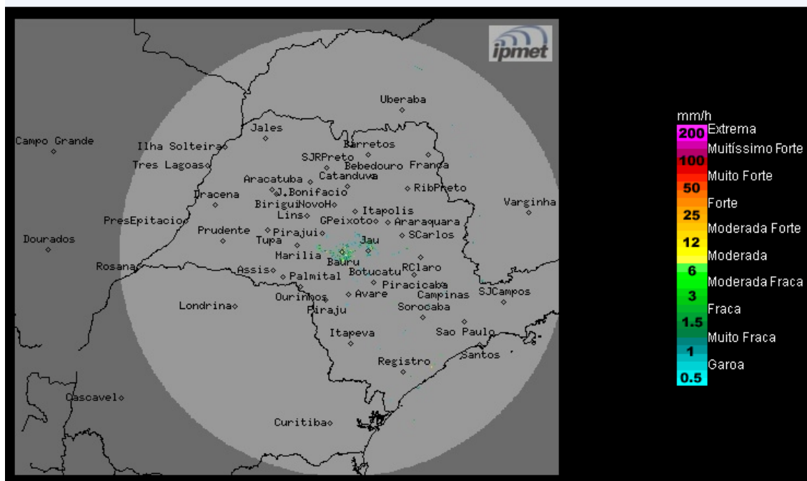
Imagem Composta dos Radares de Bauru e de Presidente Prudente - 20/07/2022 08:00
