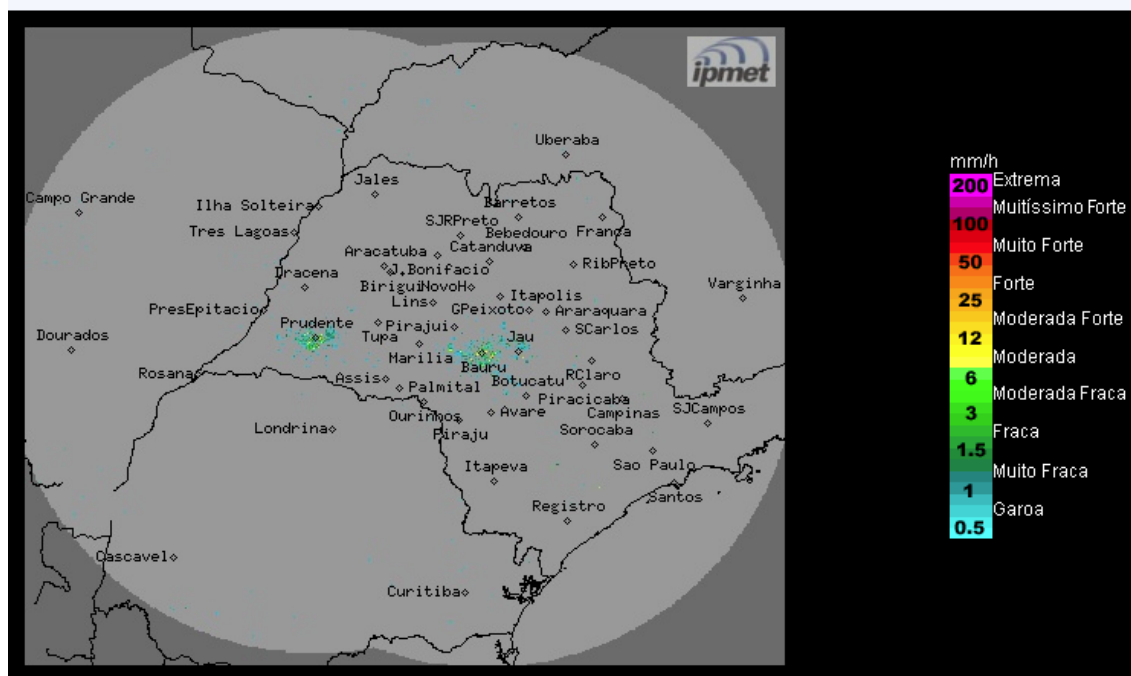
Imagem Composta dos Radares de Bauru e de Presidente Prudente - 27/12/2023 08:00
